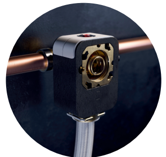
Sandwich-Anschlussarmatur der NeoSoft Lock Connect Weichwasseranlagen
